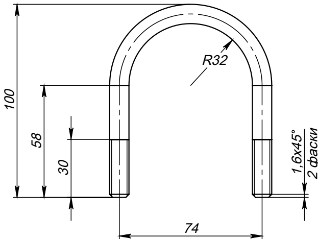
Поз.4 (Хомут)
