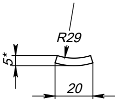
Поз.6 (Упор)
