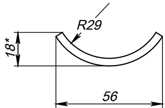
Поз.3 (Ложемент)
